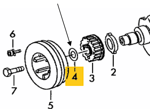
rys. 2 Pozycja montażu
